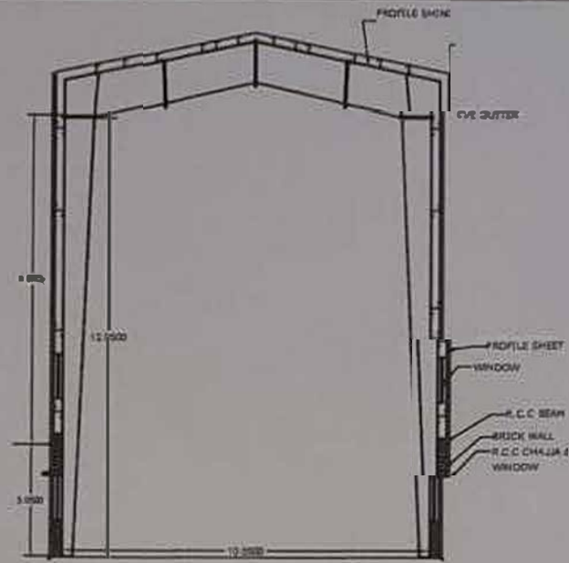
SECTION A-A
